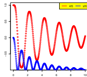
Metodo di Eulero Implicito h=0.025
