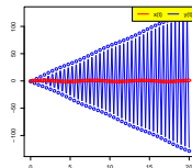
Metodo di Crank-Nicolson h=0.25
