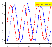
Crank-Nicolson Stabilizzato h=0.5 \tau=1
