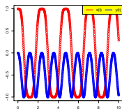
Crank-Nicolson stabilizzato
