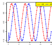
Metodo di Eulero Implicito h=0.25
