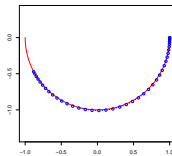
Metodo di Eulero Implicito h=0.025
