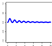
Primo vincolo nascosto h=0.025
