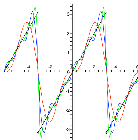
Serie di Fourier N = 2, 5, 10
